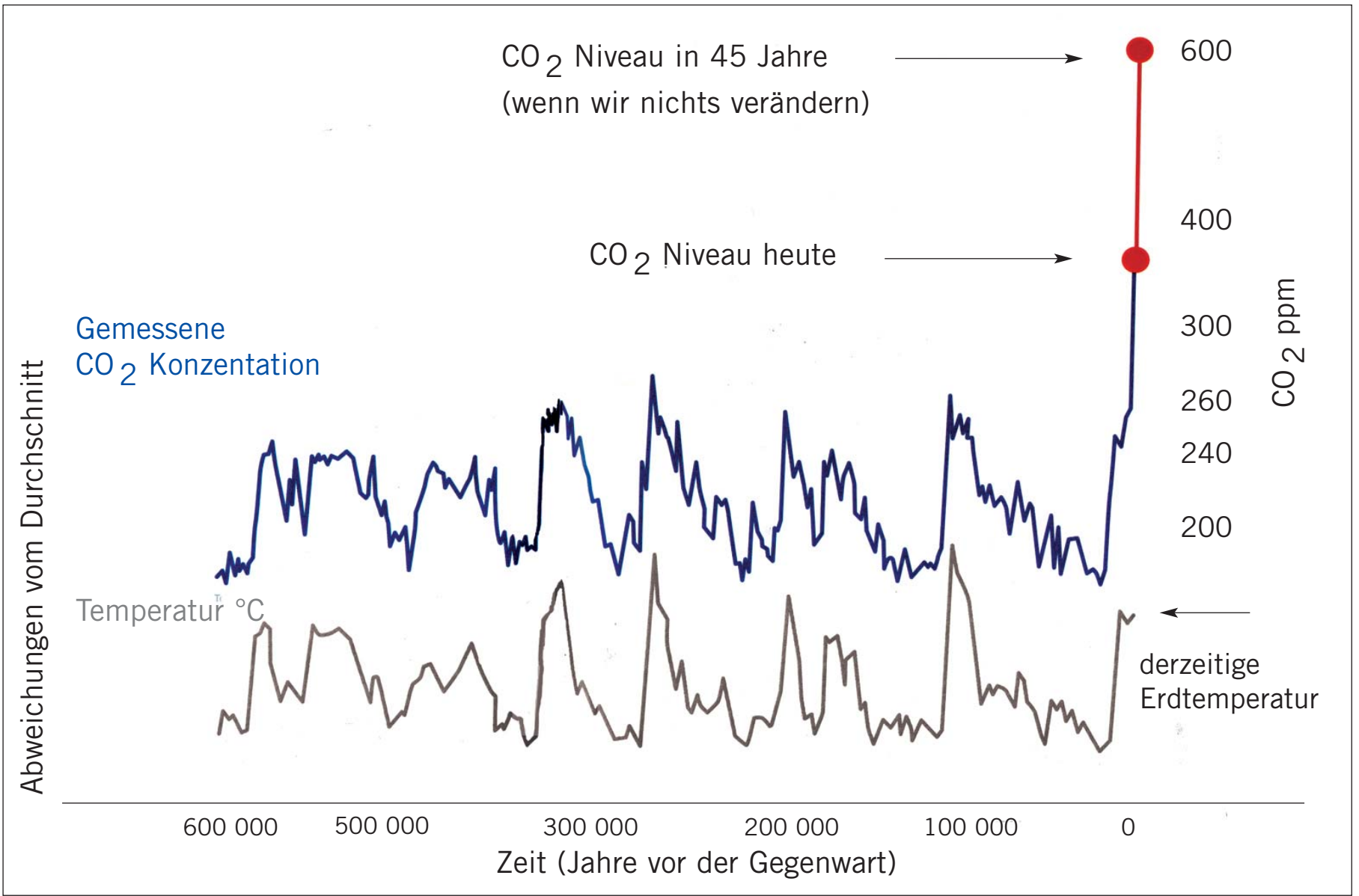
In den letzten 600.000 Jahren war die CO 2 -Konzentration noch nie so hoch wie heute
